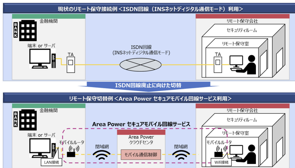
図3 リモート保守イメージ図
